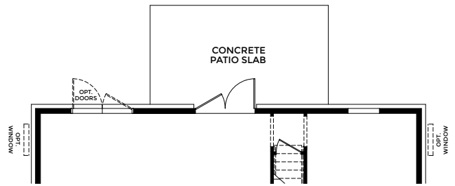
OPTIONAL 18X10 PATIO SLAB
