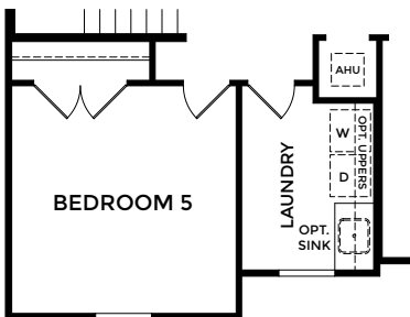
OPTIONAL BEDROOM 5
